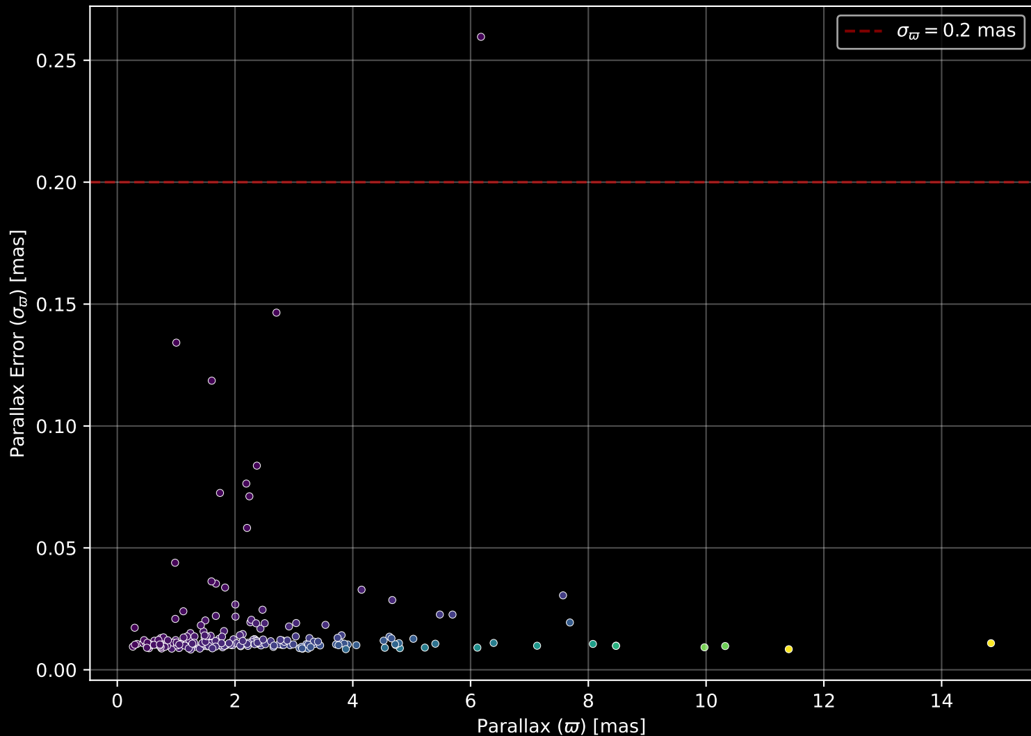
GALAH DR4 Field: [7223] Parallax Quality (n= 219)
