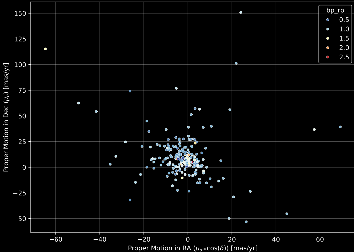
GALAH DR4 Field: [7223] Proper Motion Diagram (n= 219)
