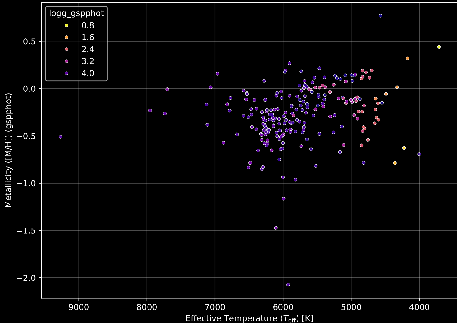
GALAH DR4 Field: [7223] Stellar Population Parameters (n= 219)
