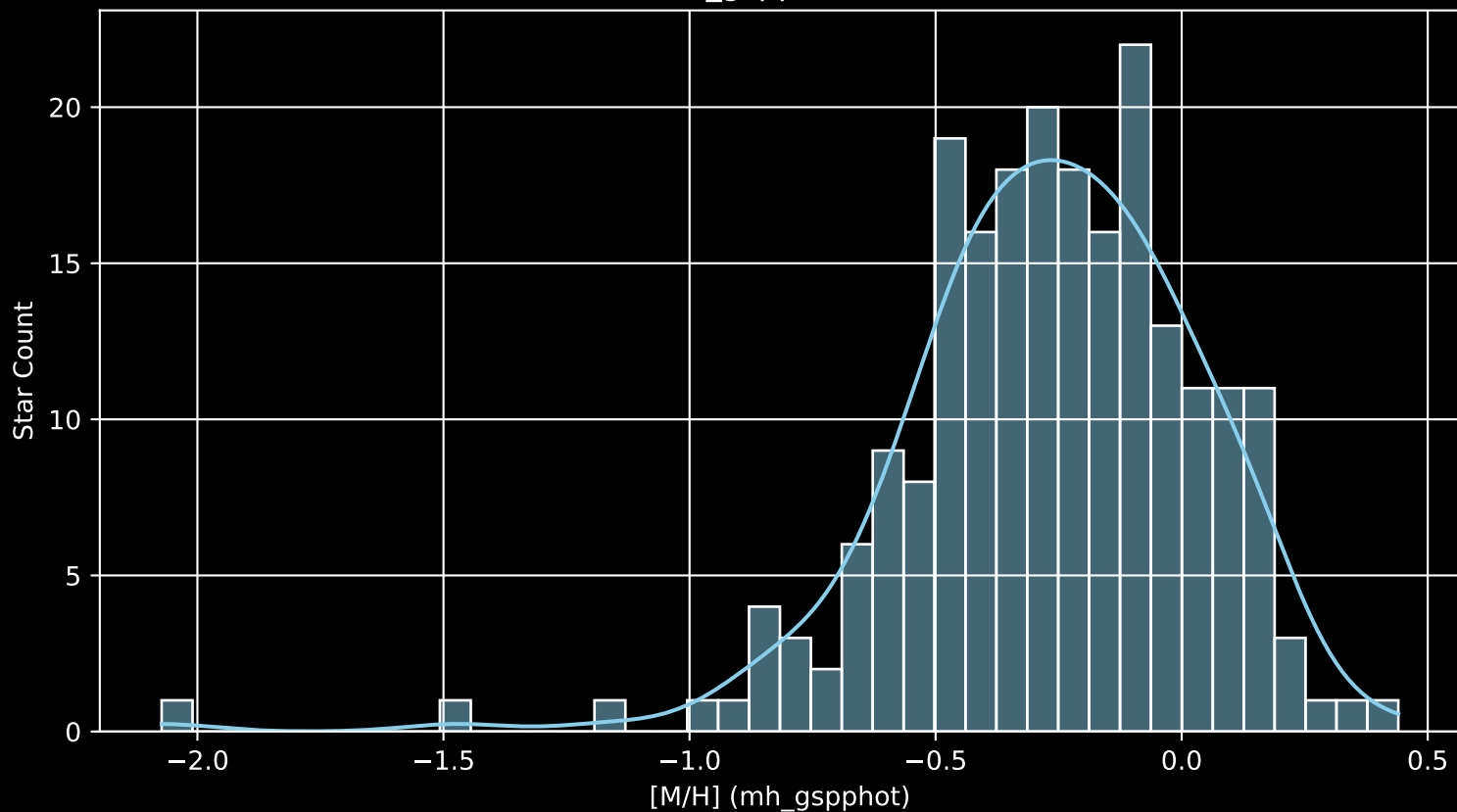
GALAH DR4 Field: [7223] [M/H] (mh_gspphot) (n= 218)
